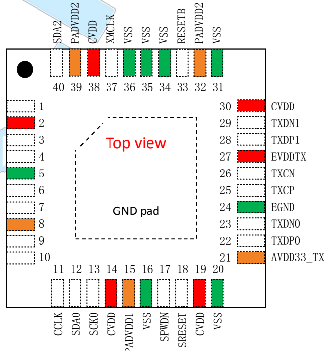
图 1 XC7022 引脚分布(俯视图)及标记图
