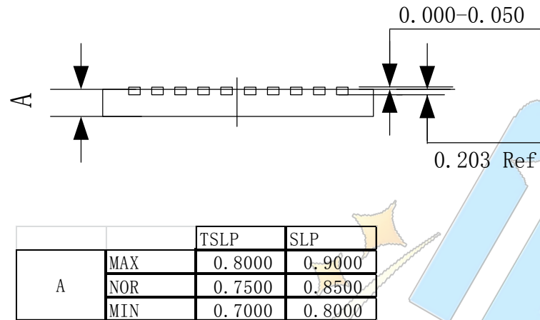
图 13 XC7022 封装侧视图
